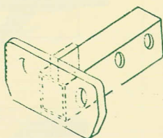
ADAPTATEUR EN D Permet transformer la rotule R en rotule standard
